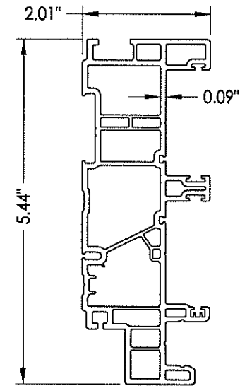
34 FRAME JAMB
