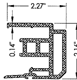
52 INTERLOCK
